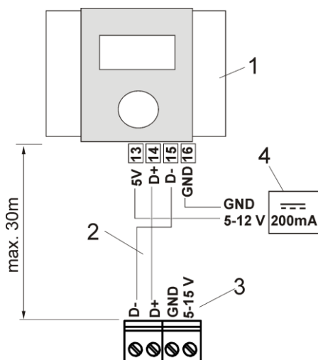
Podłączenie panelu pokojowego ecoSTER – dwużyłowe, gdzie: 1 – ecoSTER 200, 2 – przewody, 3 – ecoMAX, 4 – zasilacz 9V min 200mA.
